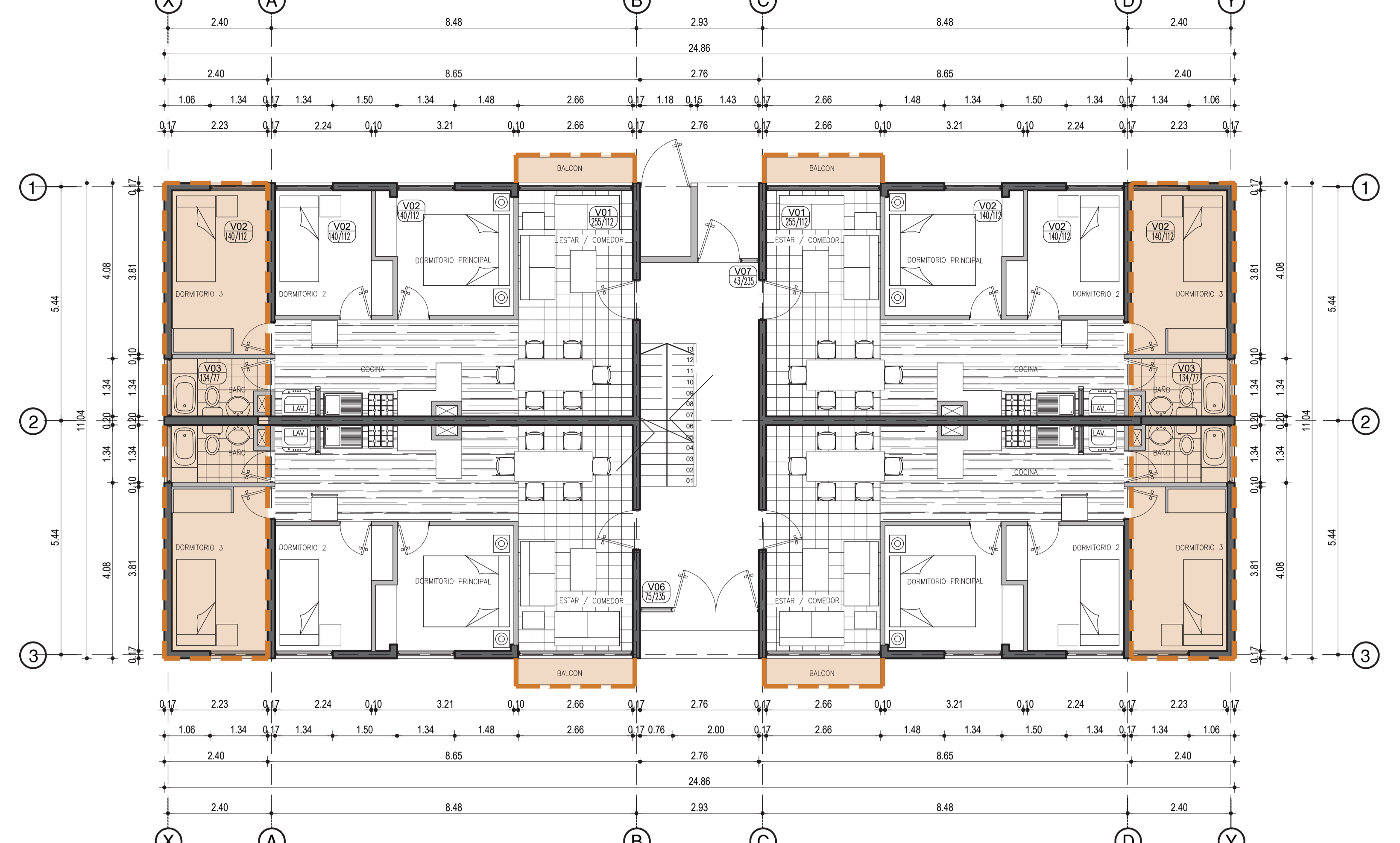
PLANTA PRIMER PISO
