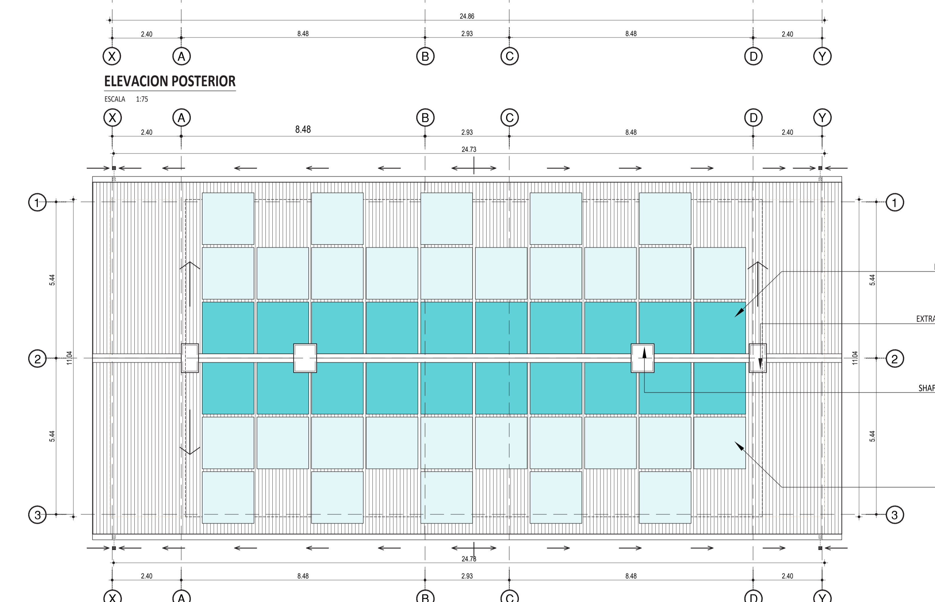
ELEVACION TECHUMBRE
