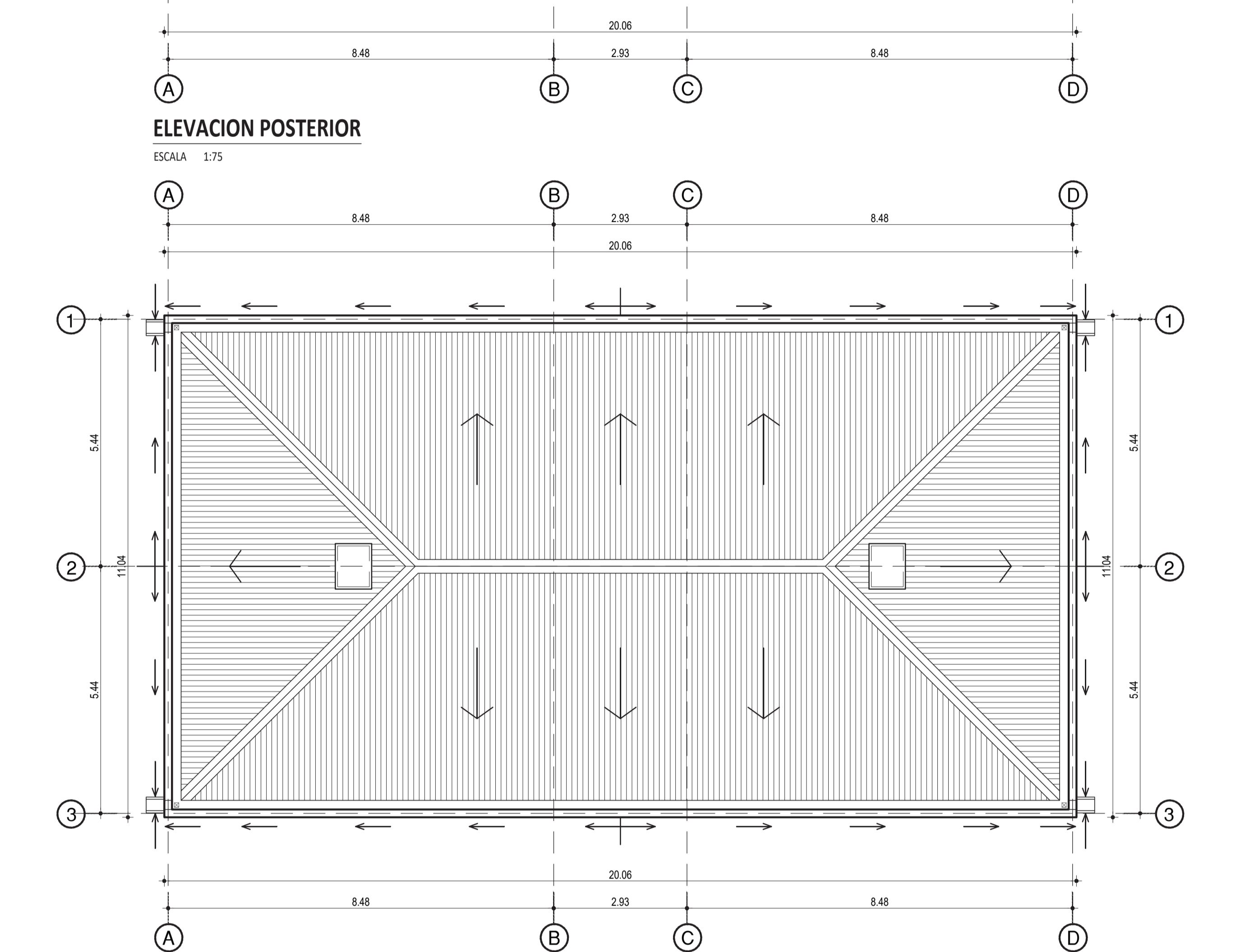
ELEVACION TECHUMBRE
