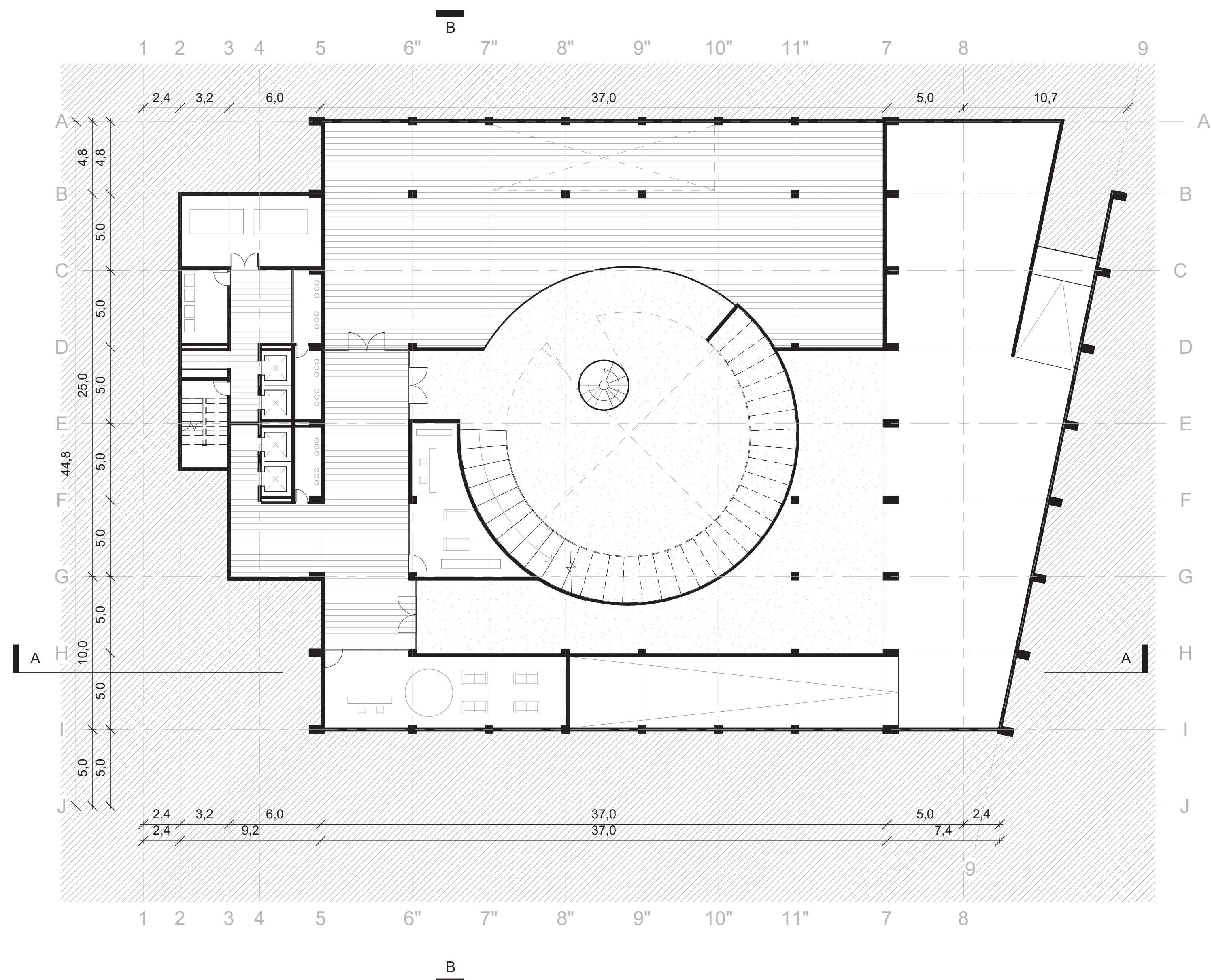
Planta Piso 2 Escala 1:200
