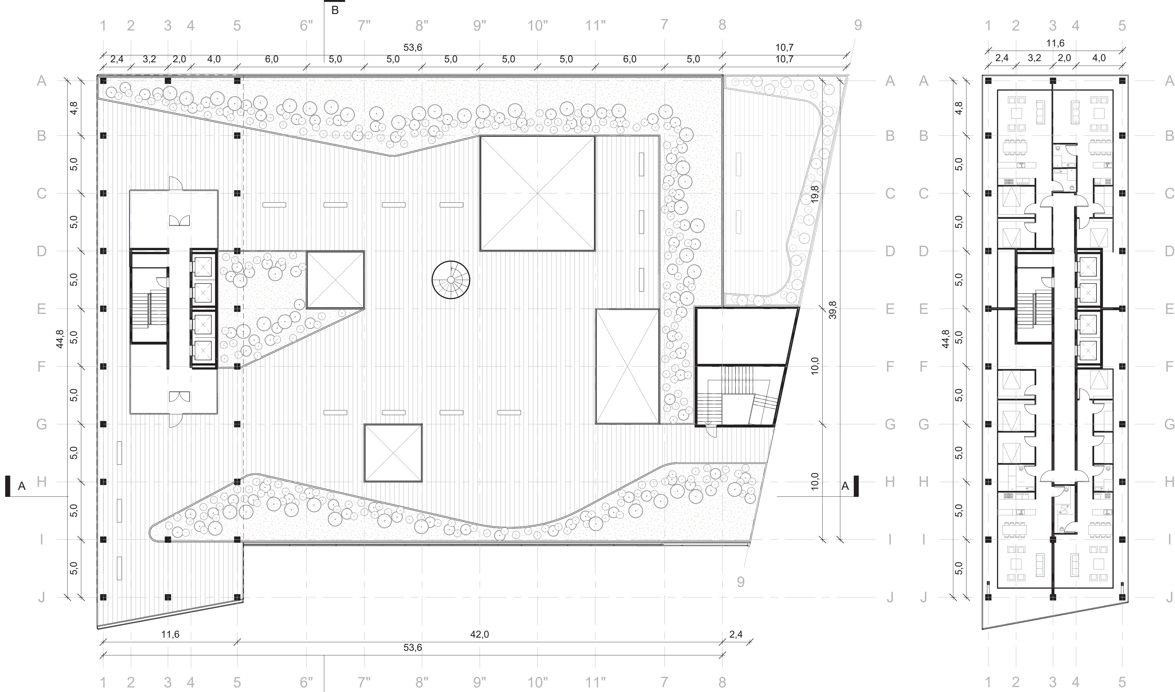
Planta Piso 5 y 6 Escala 1:200
