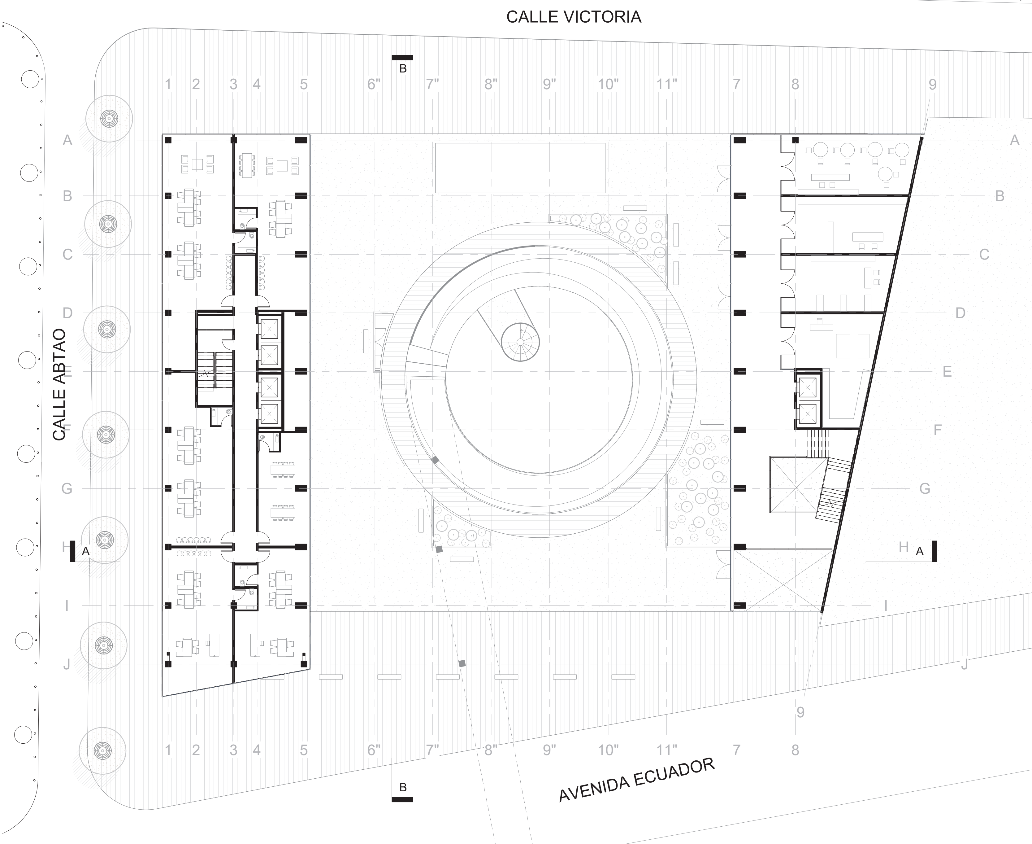
Planta Piso 4 Escala 1:200
