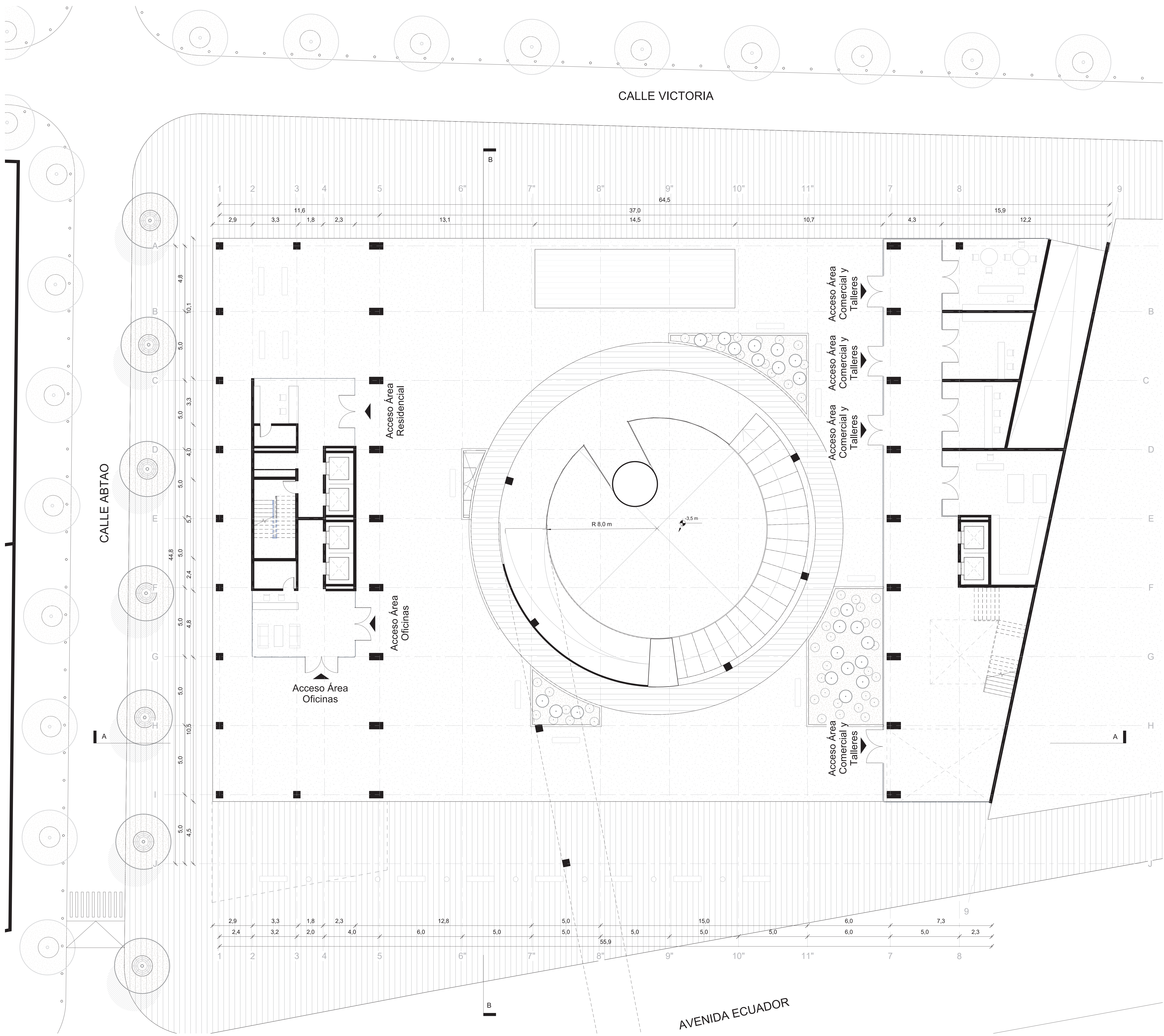
Planta Primer Piso Escala 1:100
