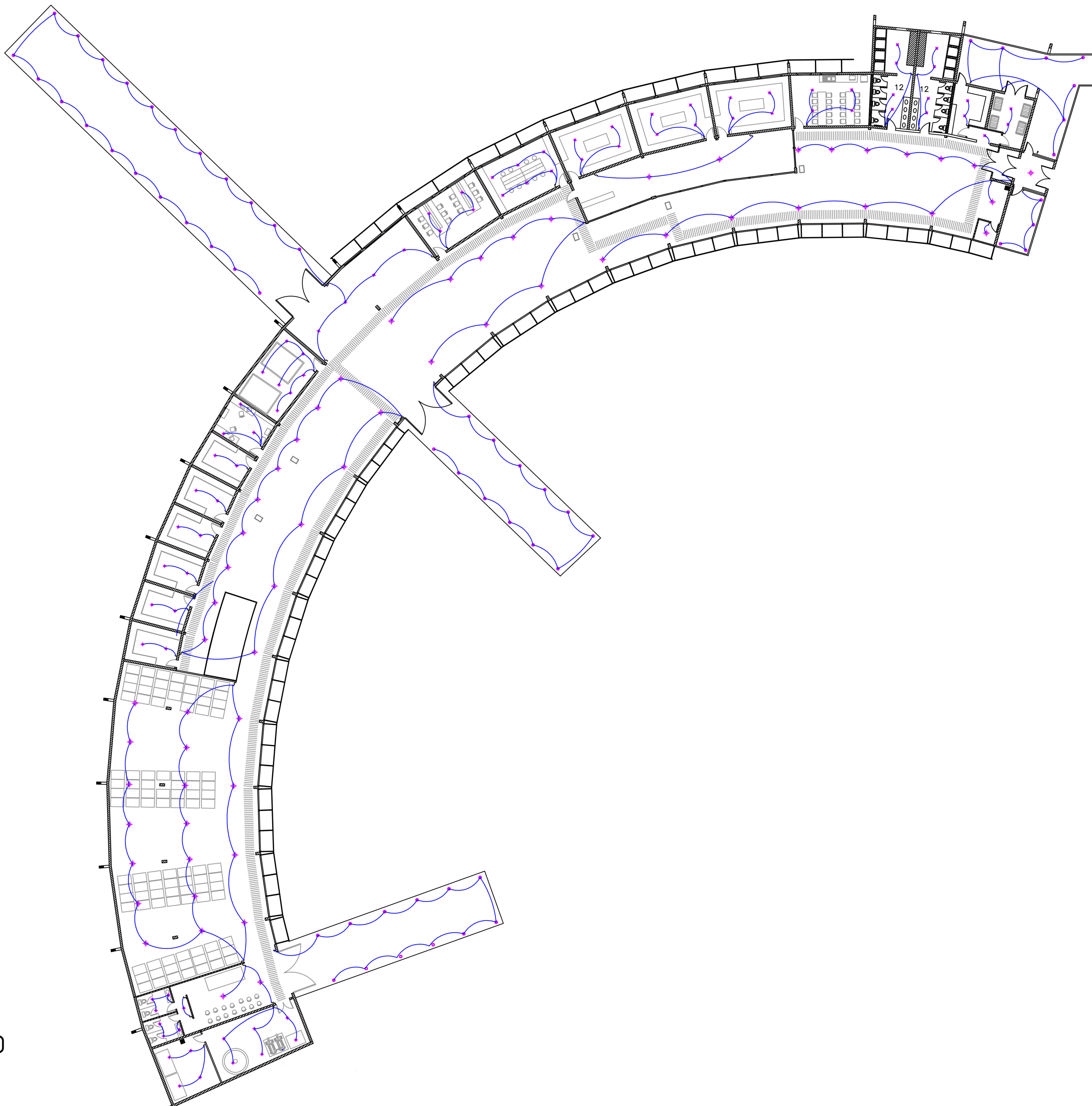
PLANO ELÉCTRICO ESC 1:250
