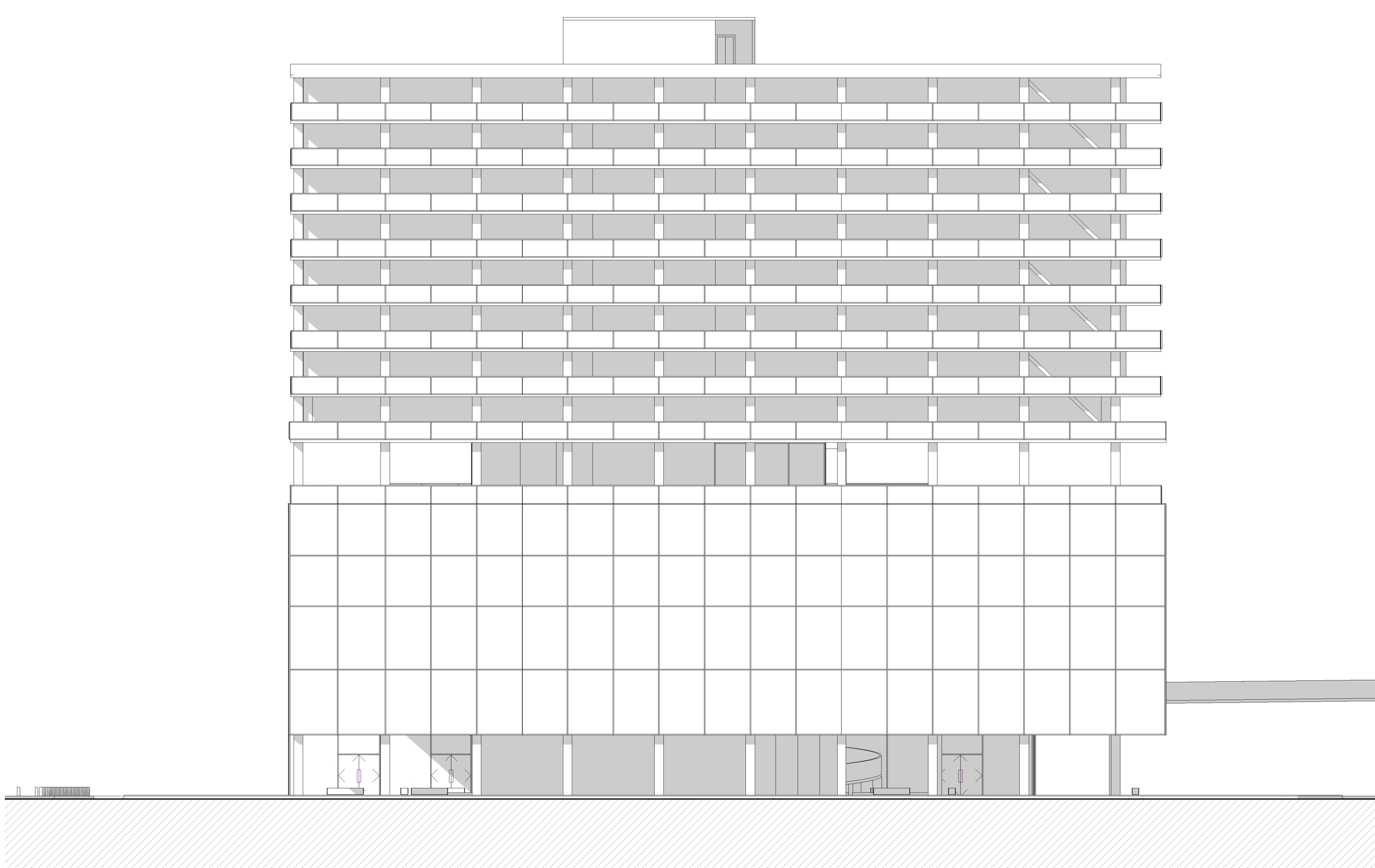
Elevación Poniente Escala 1:200
