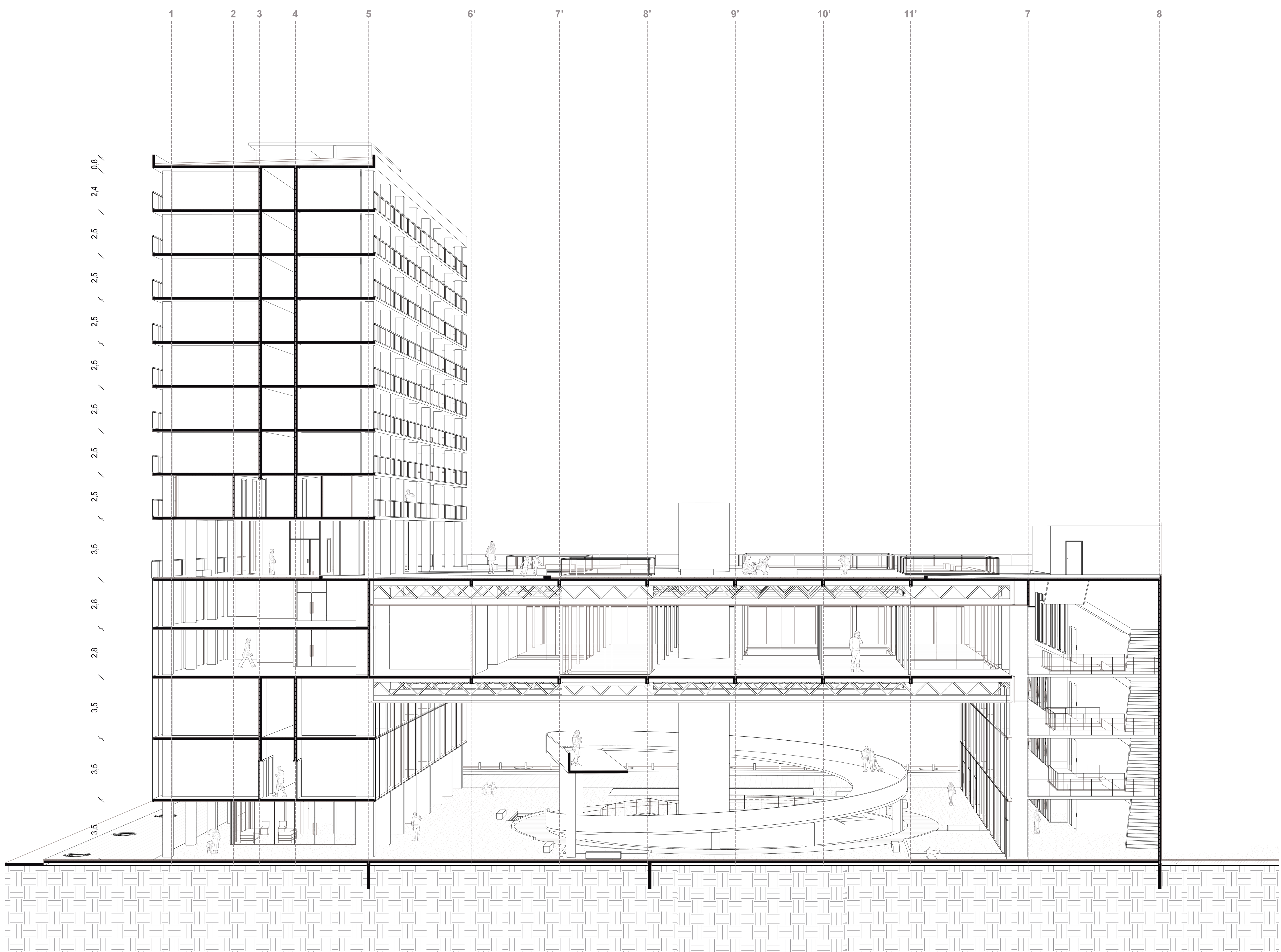
Corte Perspectivado A-A' Escala 1:100
