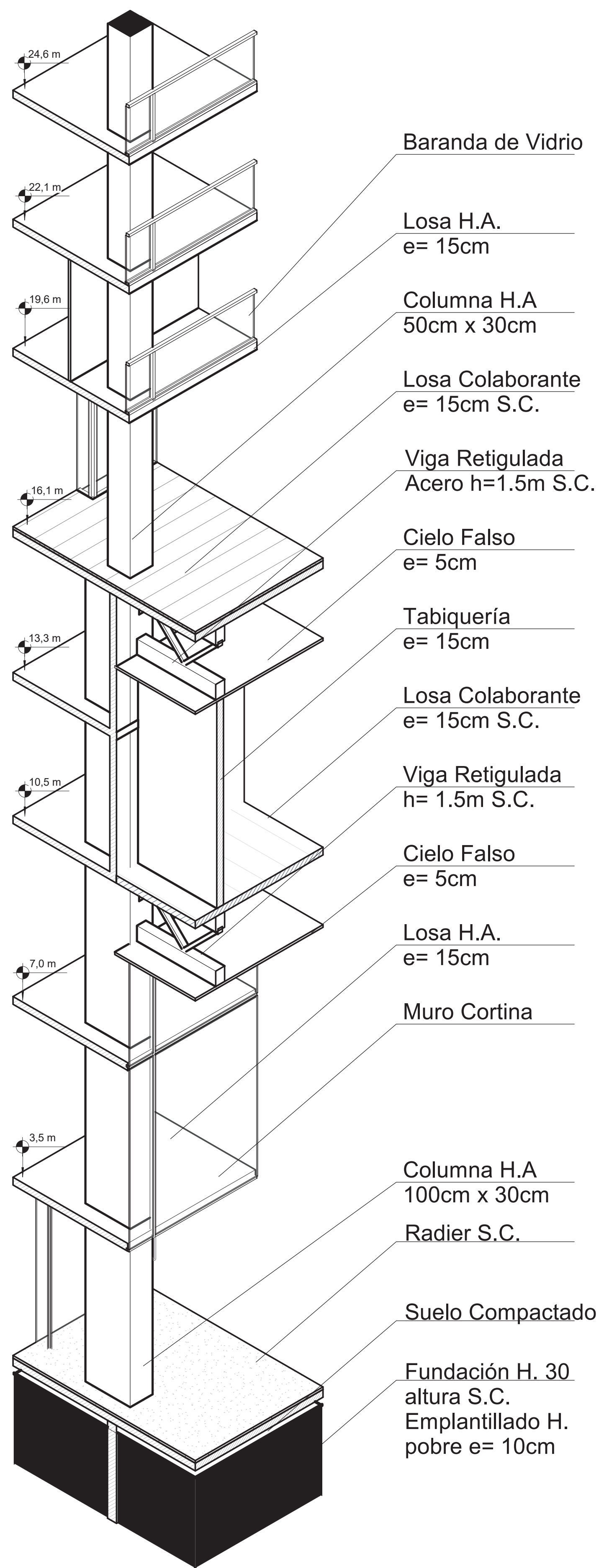
Escantillón Escala 1:30
