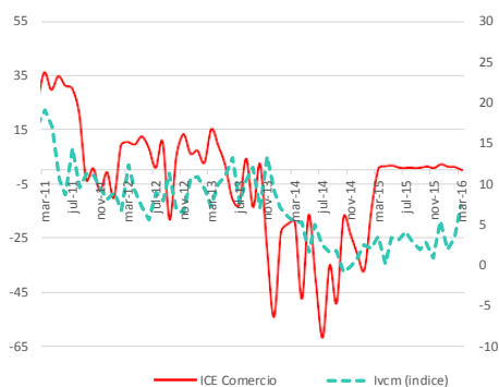
Gráfico 4 ICE Comercio e ICVM (Índice centrado en cero y variación %)
