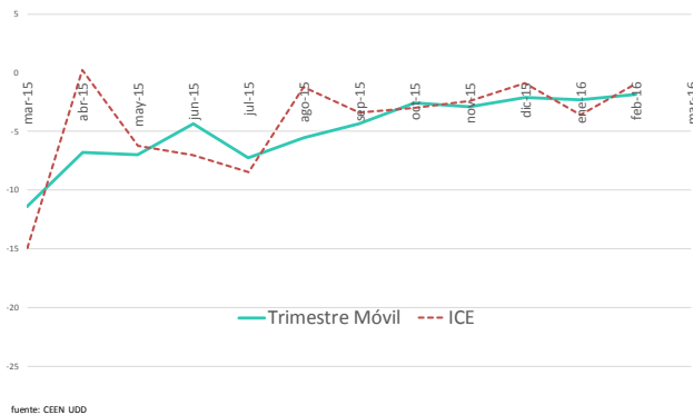
Gráfico 1.2 Trimestre móvil - ICE Marzo 2015 - Marzo 2016 (Índice centrado en cero)
