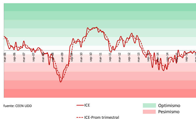
Gráfico 1.1 Trimestre móvil - ICE Marzo 2006 - Marzo 2016 (Índice centrado en cero)
