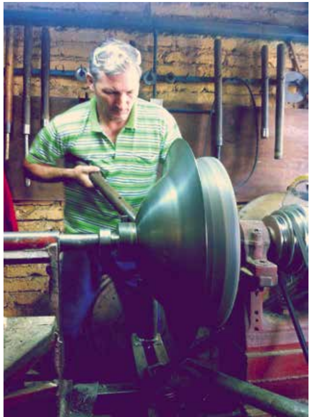
Proceso y matrices de repujado, Santiago
