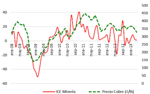
Gráfico 7 ICE Minería y Precio del cobre (Índice en base 100, eje izq y precio ¢/lb eje der)
